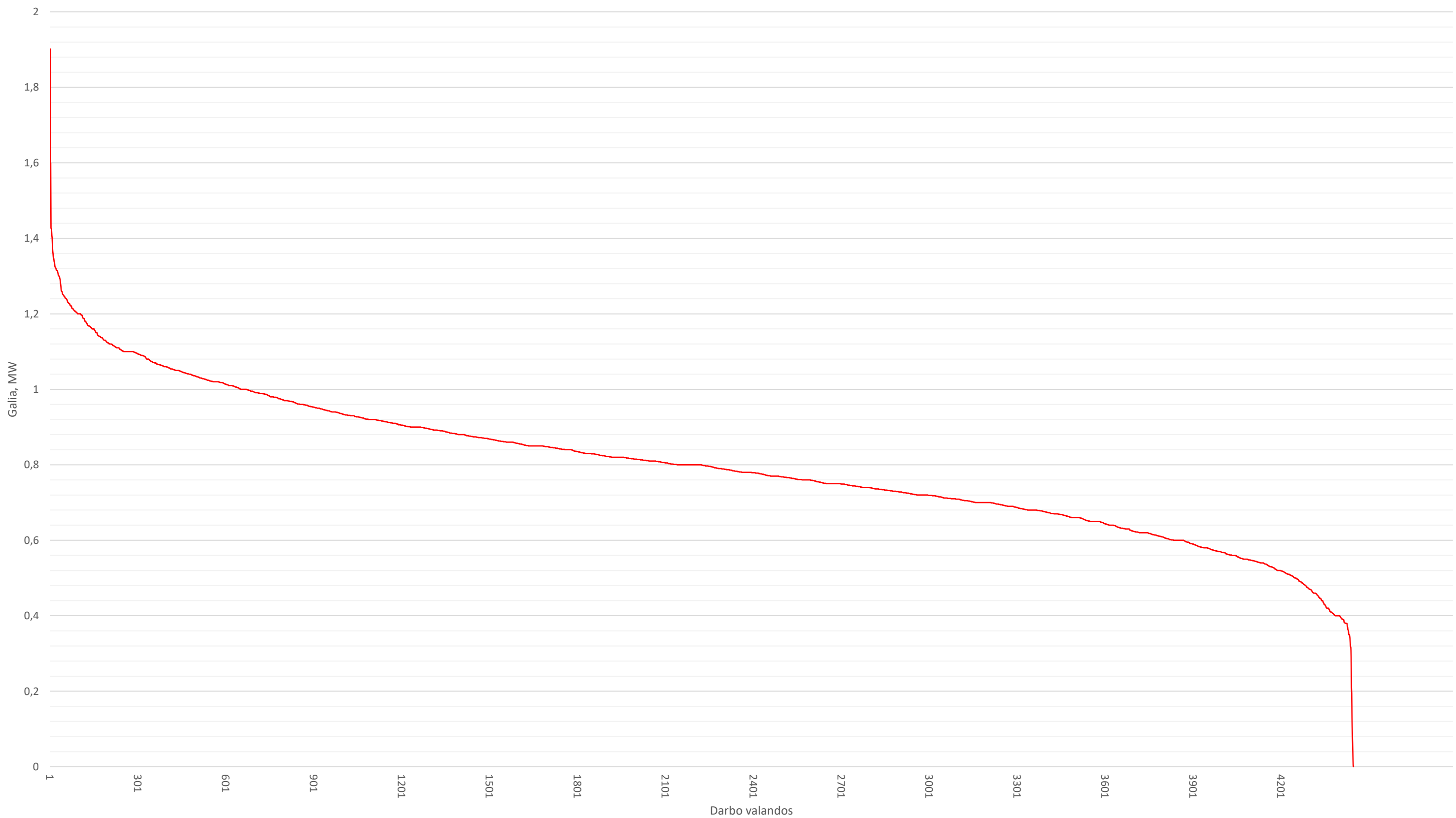
Viekšnių katilinės 2023 metų apkrovimo grafikas
