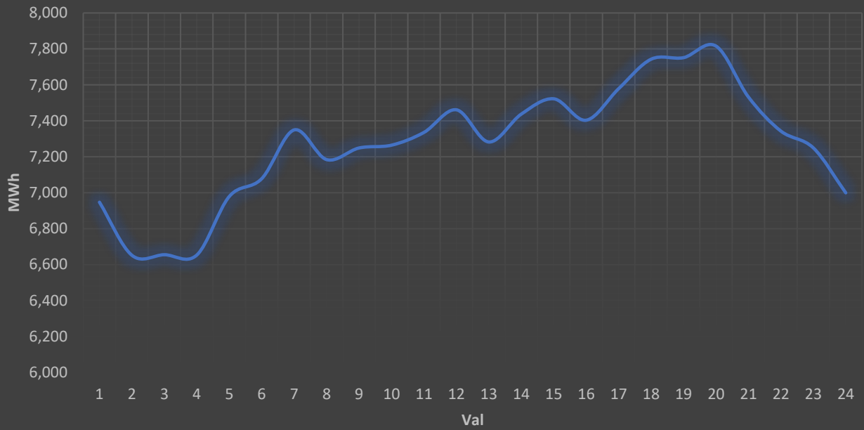
Mažeikių katilinės paros vidutinio šilumos poreikio grafikas 2025 m. nešildymo sezono metu
