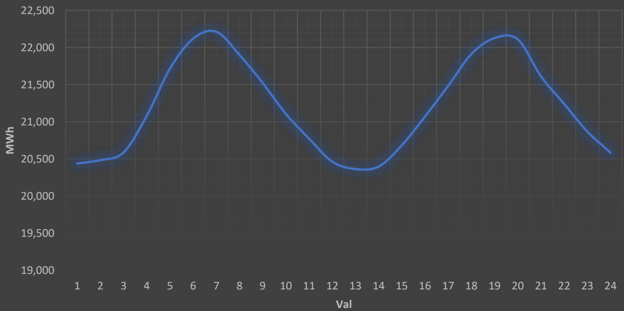
Mažeikių katilinės paros vidutinio šilumos poreikio grafikas 2025 m. šildymo sezono metu
