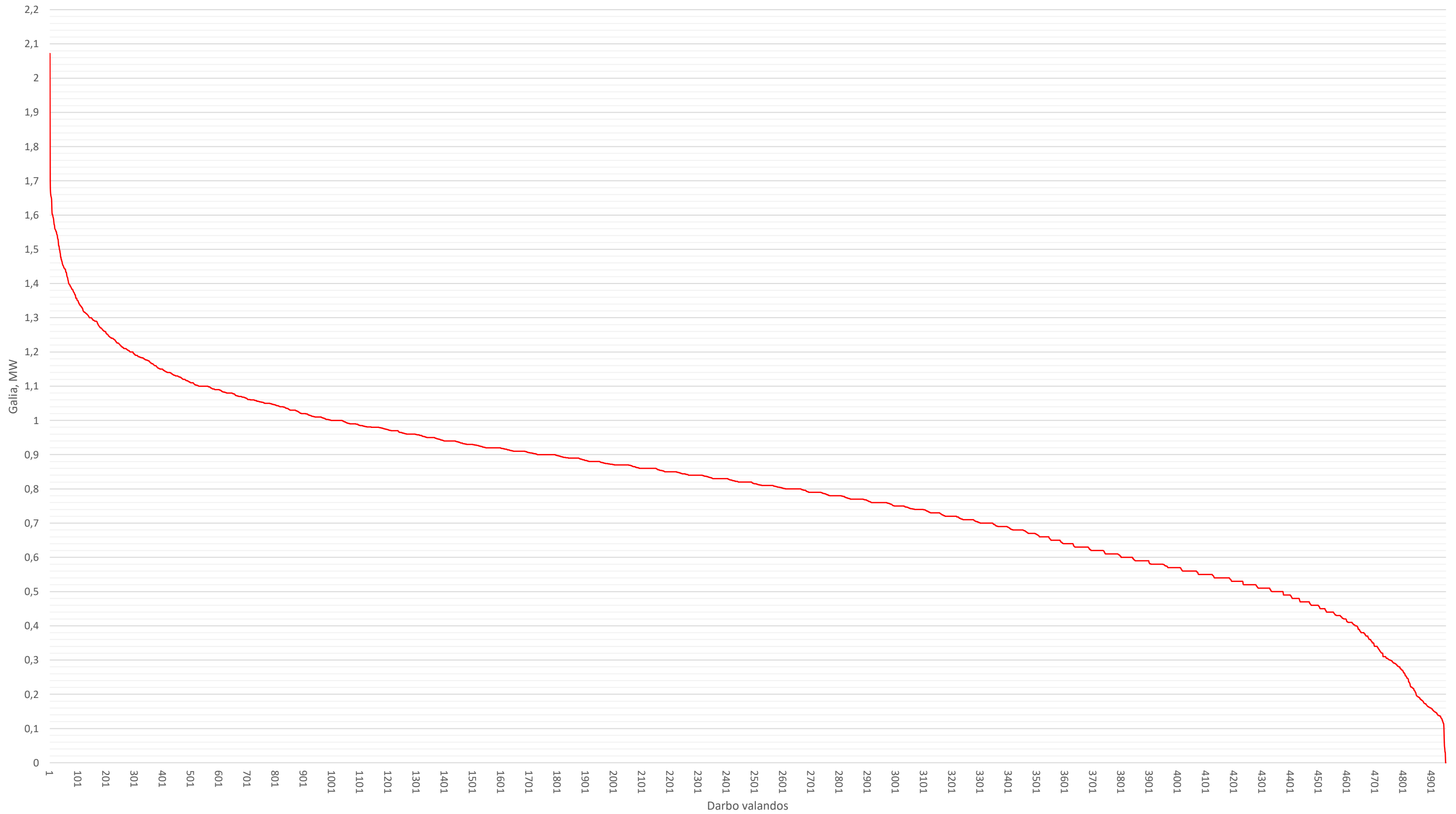
Viekšnių katilinės 2025 metų apkrovimo grafikas
